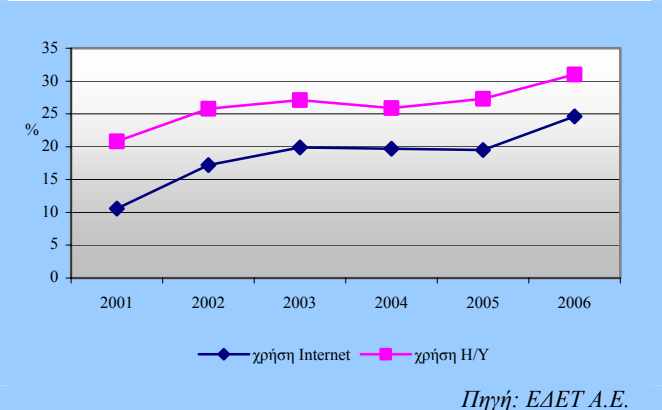
Διάγραμμα 1.1 Χρήση ηλεκτρονικού υπολογιστή και Internet στην Ελλάδα (2001-2006)
