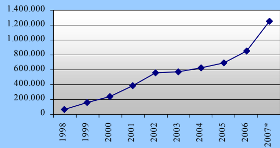
Διάγραμμα 4.1 Διαχρονική εξέλιξη του αριθμού των συνδρομητών Internet (1998-2007*)
