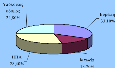
Διάγραμμα 5.1 Κατανομή παγκόσμιας αγοράς πληροφορικής και τηλεπικοινωνιών (2007)
