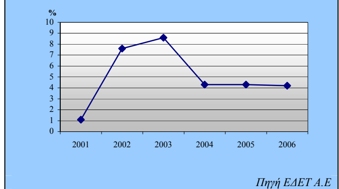
Διάγραμμα 1.4 Πρόθεση απόκτησης σύνδεσης Internet στο νοικοκυριό (2001-2006)
