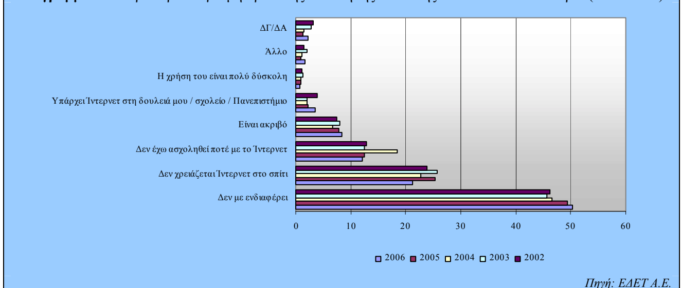
Διάγραμμα 1.5 Κυριότεροι λόγοι μη πρόθεσης απόκτησης σύνδεσης Internet στο νοικοκυριό (2002-2006)
