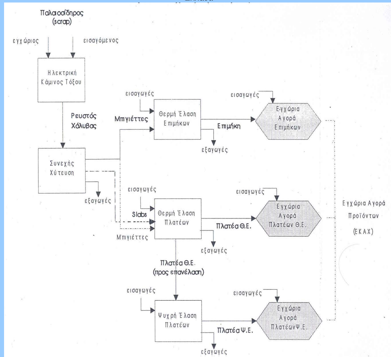
Διάγραμμα 1.1 Κύκλωμα πρώτων υλών, ημιπροϊόντων και ετοιμών προϊόντων χάλυβα (ΕΚΑΧ) στην Ελλάδα
