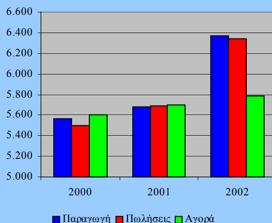
Διάγραμμα 5.3 Εξέλιξη της παραγωγής, των πωλήσεων και της αγοράς χλωριούχου πολυβινυλίου (PVC) στις χώρες της Δυτικής Ευρώπης (2000-2002)
