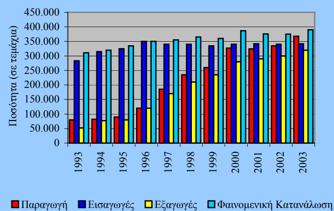
Διάγραμμα 4.1 Εγχώρια φαινομενική κατανάλωση ψυγείων-ψυγείοκαταψυκτών-καταψυκτών (1993-2003)
